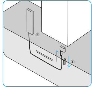
Abb. 3 Einfache Montage des Receivers Der Receiver lässt sich ohne zusätzliches Werkzeug einfach montieren: Schräge vom vorn öffnen, Stick (1) an der Innenseite der Haube entfernen und den Receiver (4) einstecken.
