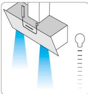
Fig. 2 El control opcional para las funciones de iluminación adicionales se instala fácilmente. El montaje de un receptor (número de pedido BLZ 501) y el acoplamiento con el control remoto (orden número 502 BLZ) permiten el control de la temperatura del color y del brillo de la campana.
