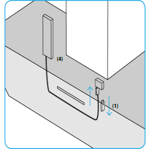
Sl. 3 Jednostavna montaža prijemnika Prijemnik se lako instalira bez dodatnih alata. Uklonite štapić (1) unutar aspiratora i postavite prijemnik (4).
