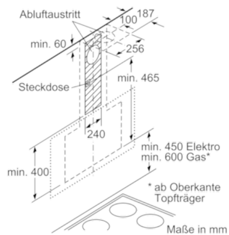
Maximale Stärke der Rückwand beachten. Maße in mm
